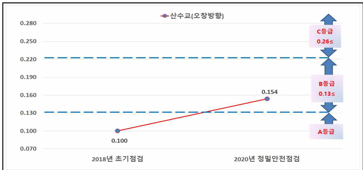
[그림 5.4.1] 산수교 오창방향 상태평가 결과 비교 그래프
